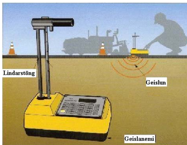
Mynd 1: Troxler tæki. Geislaálaginn mælir gammaálag og nifteindaálag sem endurvarpast úr jarðvegi.
